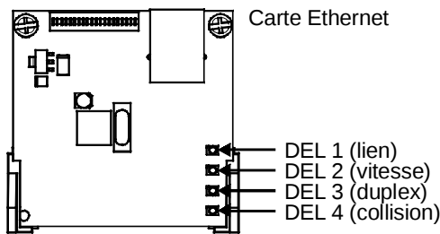
Figure 4 : Voyants DEL
